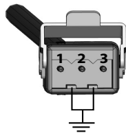
Antriebsanschluss
